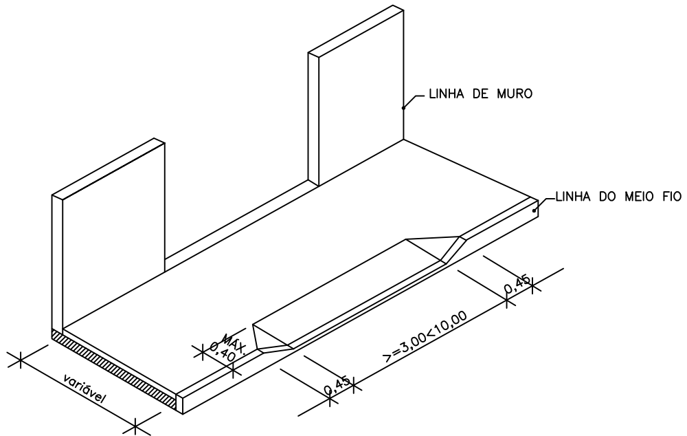
Detalhe padrão do rebaixo no passeio público para acesso de veículos.
